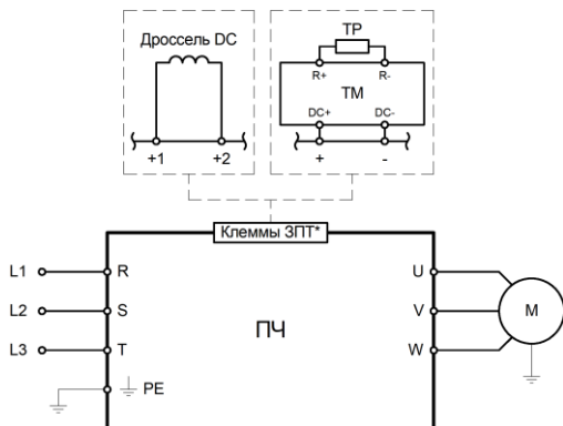
Рисунок 2ж – Подключение силовых клемм для моделей LCI-GY/PY-6
