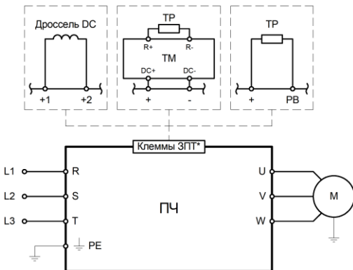
Рисунок 2д – Подключение силовых клемм для моделей LCI-GY/PY-4(B)
