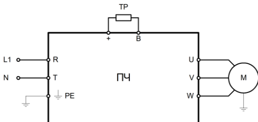
Рисунок 2в – Подключение силовых клемм для моделей LCI-GY/PY-2B (S)
