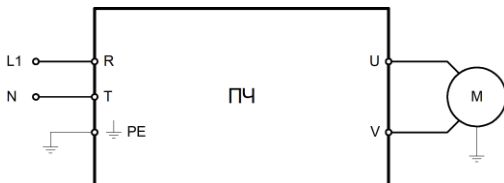
Рисунок 2а – Подключение силовых клемм для моделей LCI-GY/PY-1
