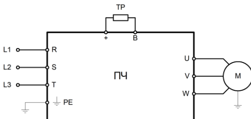
Рисунок 2е – Подключение силовых клемм для моделей LCI-GY/PY-4B (S)
