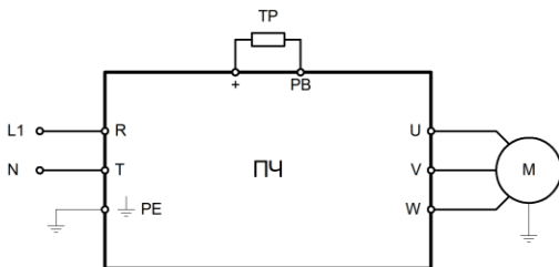
Рисунок 2б – Подключение силовых клемм для моделей LCI-GY/PY-2(B)
